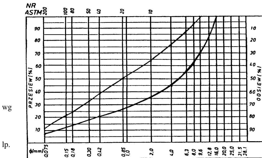
Rys. 1. Krzywe graniczne uziarnienia mieszanki mineralnej 0÷12,8 mm do warstwy ścieralnej z betonu asfaltowego dla KR 2
