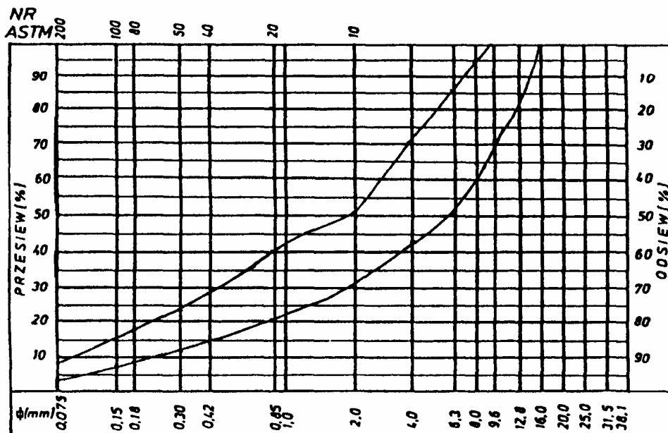
Rys. 2. Krzywe graniczne uziarnienia mieszanki mineralnej 0+16 mm do warstwy wiążącej, wyrównawczej i wzmacniającej z betonu asfaltowego dla KR 2
